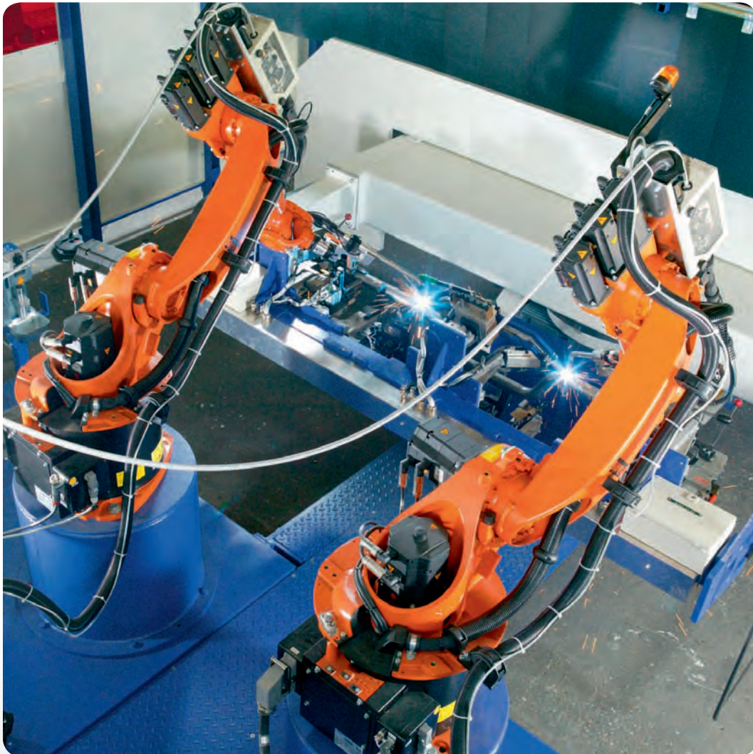
Roboter-MAG-Schweißen von Rohrkörpern mit zwei Robotern und 180 Grad reversierendem Drehtisch
